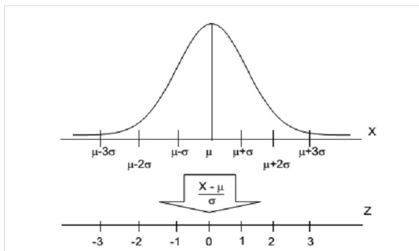
Figura A6-2 - Distribuição Normal típica normalizada
